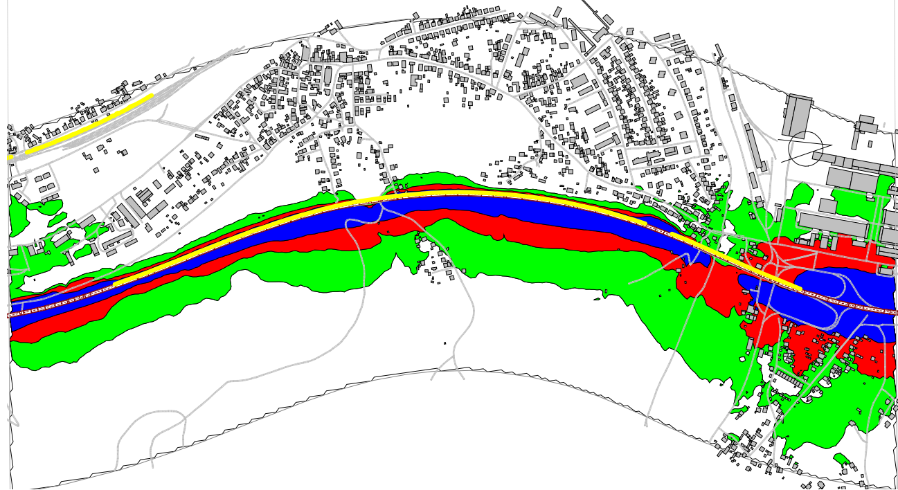
Konfliktný plán po realizácii PHC
