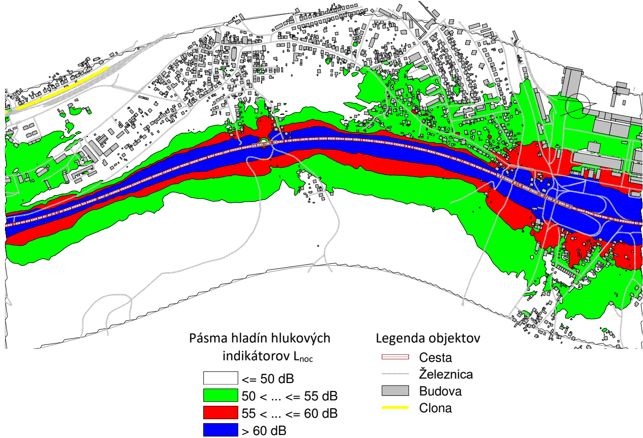
Konfliktný plán pred realizáciou PHC
